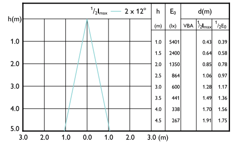
LEDspots 14W PAR38 E26 927 25D
