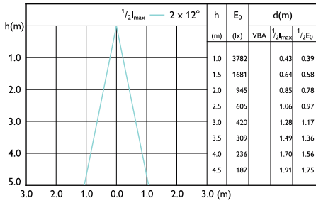
LEDspots 10W PAR38 E26 930 25D
