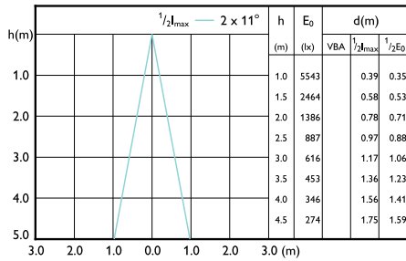
LEDspot PAR38 6,5-50W 525lm 25D 6500K E27
