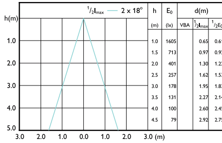
LEDspots 10W PAR38 E26 930 40D
