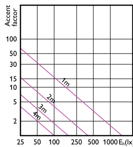
LEDspots 10W PAR38 E26 930 40D
