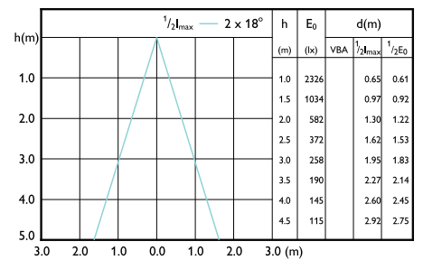
LEDspots 14W PAR38 E26 930 40D
