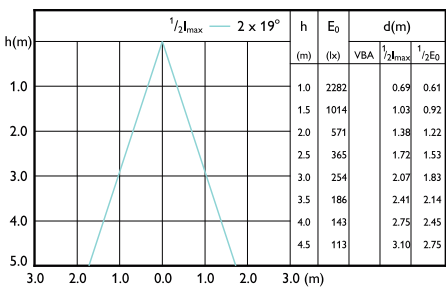
LEDspots 14W PAR38 E26 927 40D
